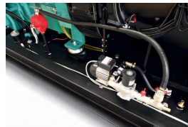
Automatisches Kraftstoffnachfüllkit Automatic refuelling device
